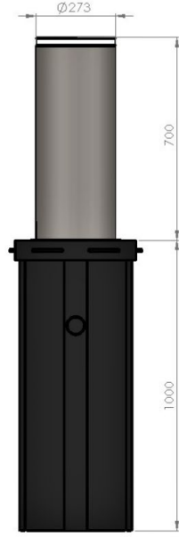
ÖN GÖRÜNÜM
