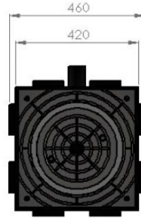
ÜST GÖRÜNÜM
