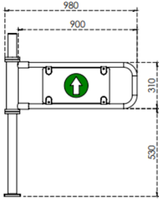
ÖN GÖRÜNÜM
